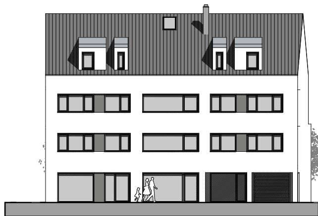
ansicht von norden haus 3
