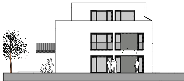
ansicht von süden haus 2
