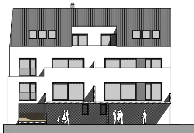
ansicht von süden haus 3
